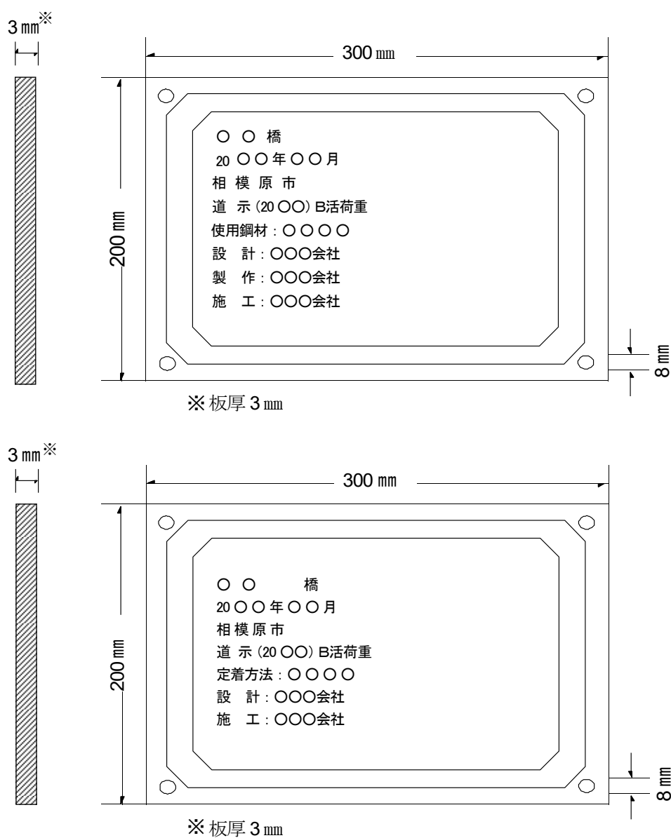
図2-2 銘板の寸法及び記載事項
