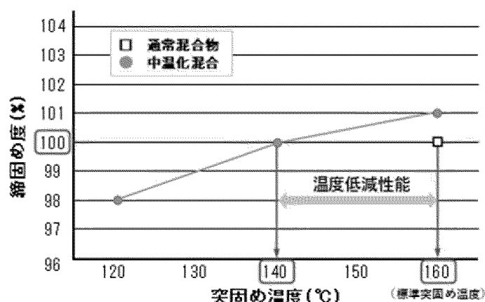
図2－6 温度－突固め度のグラフ（作成例）
