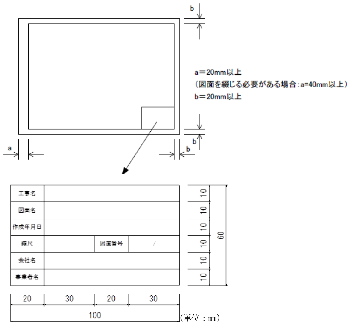
図 5-2 輪郭と余白及び表題欄
