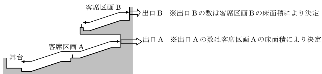
断面図
