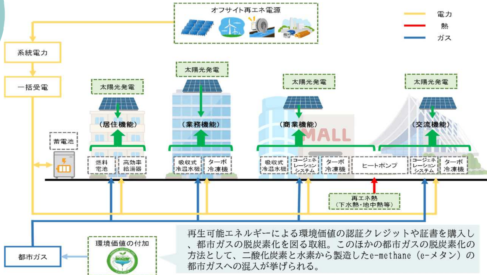
図 参考：地域エネルギーシステムの例
