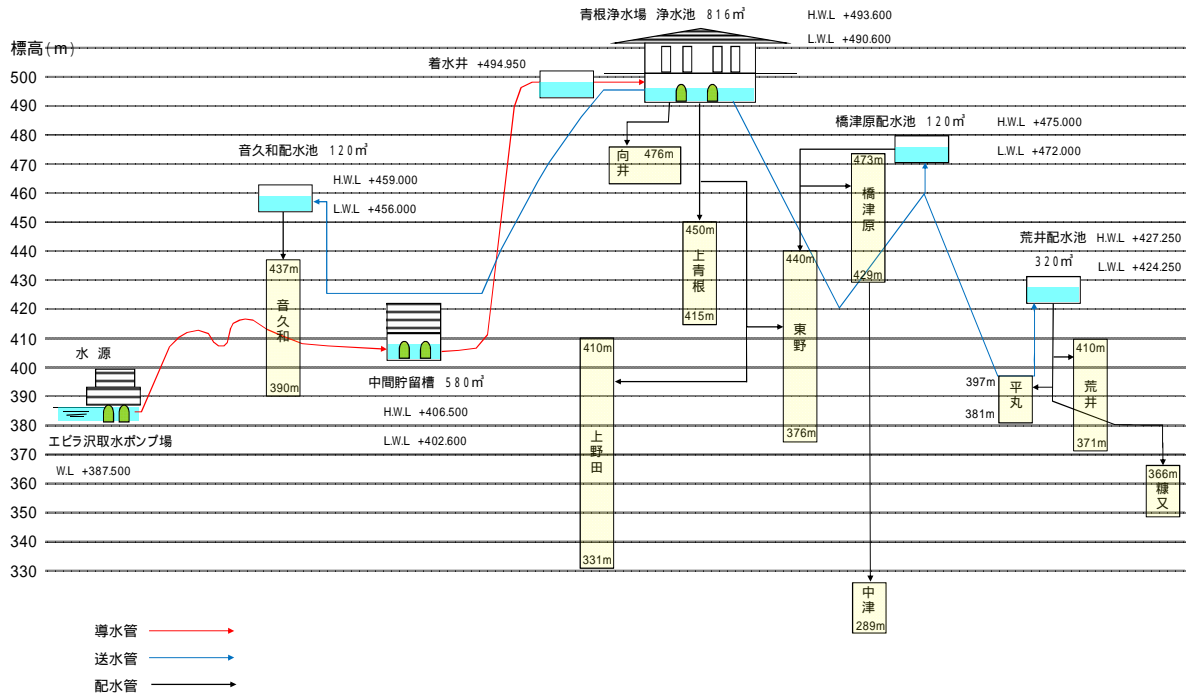
図3 給水地域図、施設縦断フロ-図
