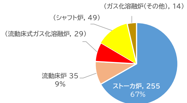
図 7.3-1 国内のごみ焼却形式(平成 30 年度)
