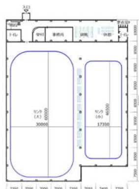
練習中心型スケートリンク（建築面積：約4,500㎡）
